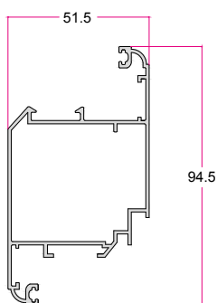
لنگه لولایی درب داخل باز شو Inside Opening Door Sash 1.200 (kg/m) v
