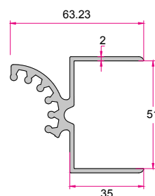
پروفیل چرخشی لوور مخصوص ۱۲۰۴ Louvre Adjustable Profile 1.240 (kg/m)
