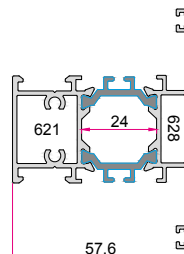
سپری سری B Series "B" Tripartalouss 1.500 (kg/m)
