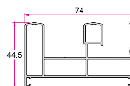
چهارچوب کشویی ساده Simple Sliding Frame 1.150 (kg/m)
