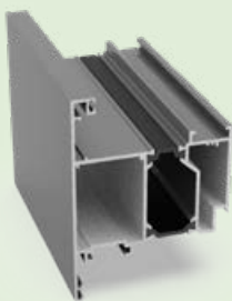
پروفیل فریم Window Frame 1.630 (kg/m)
