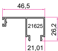
درپوش فریم مونوریل Cap for frame 0.432 kg/m
