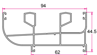
چهارچوب کشویی پهن یک طرف قوس Wide Sliding Frame 1.460 (kg/m)
