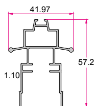
دسته توری پلیسه تیپ A Handle Profile 0.680 (kg/m)
