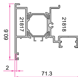
پروفیل ما بین دولنگه Outside Opening Door Sash 1.460 (kg/m)
