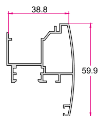
دولنگه لولایی Middle Sash 0.730 (kg/m)
