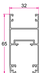
لنگه کشویی ساده کیپر دار Simple Sliding Sash 0.860 (kg/m)
