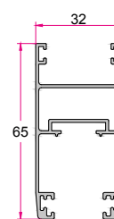
لنگه کشویی ساده کپردار Simple Sliding Sash 0.860 (kg/m)
