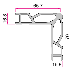
فیکس پانچی ۱۶ Corner Joint 2.200 (kg/m)
