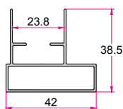
مقابل متحرک پلیسه تیپ A Fixed Sash 0.545 (kg/m)
