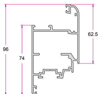
لنگه درب Door Sash 1.600 (kg/m)
