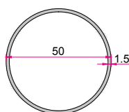
لوله ۵۰ Pipe 50 0.742 (kg/m)
