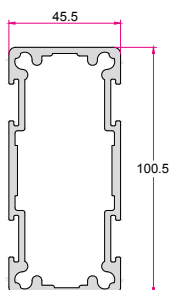
پروفیل اتصال ۱۱۰۳ Connector 2.910 (kg/m)
