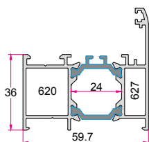
فریم کوچک سری B Series "B" Small Frame 1.400 (kg/m)
