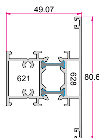
سپری سری A Series "A" Tripartalouss 1.400 (kg/m)
