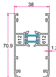
لنگه کشویی بدون زهوار Sliding Sash 1.094 (kg/m)
