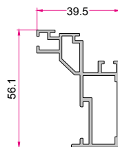
لنگه بازشو زهوارخور Opening Sash 0.800 (kg/m)
