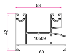
فریم Frame 1.022 (kg/m)
