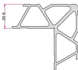
فیکس پانچی ۳۰ Corner Joint 2.800 (kg/m)
