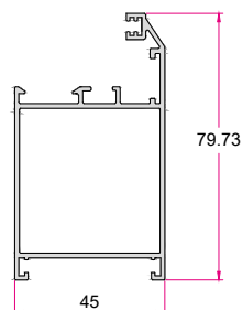
چهارچوب لولایی فولکس واگن Frame 0.998 (kg/m)
