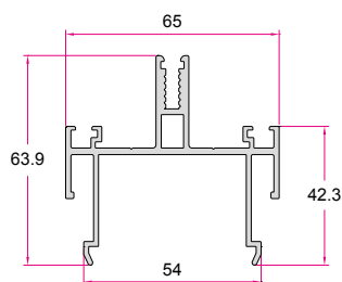
پروفیل عمودی Mullion 1.475 (kg/m)
