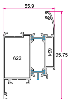
لنگه درب سری A Series "A" Door Sash 1.650 (kg/m)
