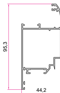
لنگه لولایی پنجره Window Frame 1.010 (kg/m)
