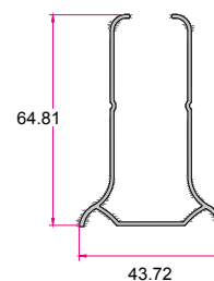
شیشه گیر Glass Clip Profile 0.650 (kg/m)
