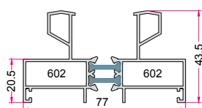
چهارچوب کشویی بدون ریل توری Sliding Frame 1.290 (kg/m)
