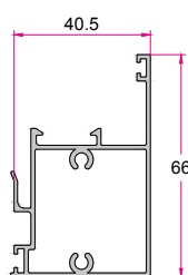
مکمل Complement Frame 0.854 (kg/m)
