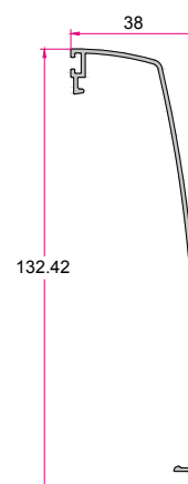
قاب Cladding 0.390 (kg/m)
