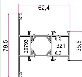
وادار لیفت اند اسلاید Tripetalous Profiles 1.550 kg/m
