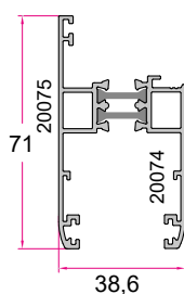
لنگه ی بازشو کشویی Vent profile 1.055 kg/m
