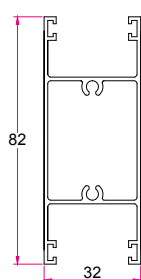
وا دار وسط کشویی Mullion 0.940 (kg/m)
