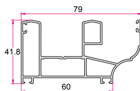
چهارچوب کشویی طرح‌دار لاستیک‌خور Sliding Frame with Rubber Place 1.100 (kg/m)
