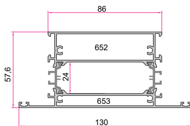
وادر پهن TH60 Tripetalous TH60 1.885 (kg/m)
