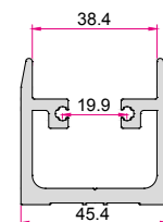
لقمه سنگین Transom 1.635 (kg/m)
