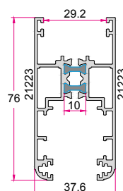
لنگه کشویی بدون زهوار Sliding Sash 1.385 (kg/m)
