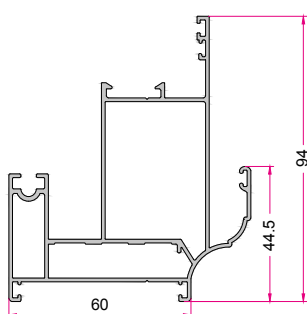
چهارچوب Monorail Frame 1.750 (kg/m)
