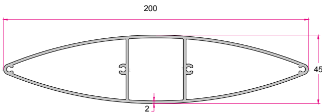
لوور ۲۰ 20cm Oval Louvre 2.580 (kg/m)
