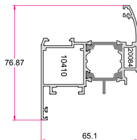
لنگه پنجره Window Sash 1.520 (kg/m)
