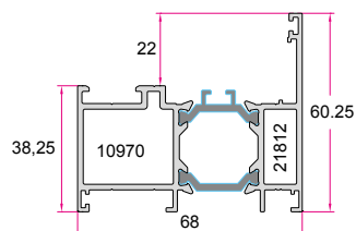
پروفیل فریم Window Frame 1.630 (kg/m)
