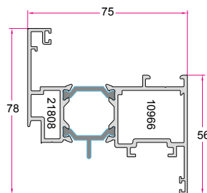
لنگه پنجره Window Sash 1.780 (kg/m)
