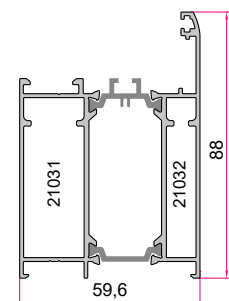
فریم فولکس واگن TH60 TH60 Frame 1.781 (kg/m)
