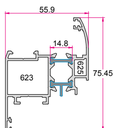
لنگه پنجره سری A Series "A" Window Sash 1.400 (kg/m)
