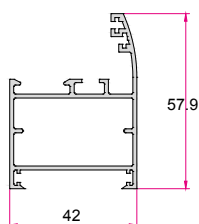
چهارچوب لولایی پنجره ۴۲ Window Frame 0.766 (kg/m)
