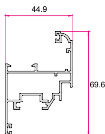
لنگه پنجره یراق پی وی سی خور Window Sash with PVC Fitting 0.940 (kg/m)
