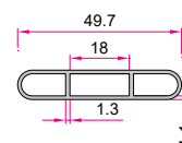
گریل Grill 0.349 (kg/m)
