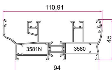
چهارچوب کشویی Sliding Frame 1.700 kg/m
