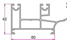
فریم Frame 1.280 (kg/m)
