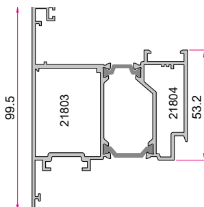
لنگه درب بیرون بازشو Between Two Sash Profile 2.390 (kg/m)
