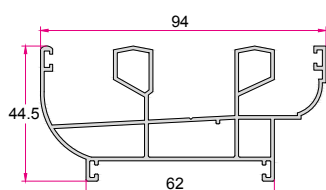
چهارچوب کشویی پهن دو طرف قوس Wide Sliding Frame 1.460 (kg/m)
