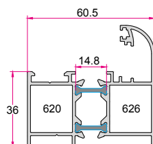
فریم متوسط سری A Series "A" Medium Frame 1.400 (kg/m)
