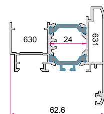
وسط دولنگه سری B Series "B" Middle Sash 1.300 (kg/m)
