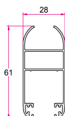
لنگه کشویی تک جداره ۶۱ سری ۵۵ Series 55 Single-Glazing Sash (6cm) 0.695 (kg/m)
