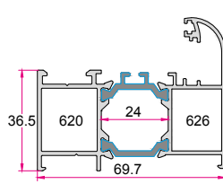
فریم متوسط سری B Series "B" Medium Frame 1.500 (kg/m)
