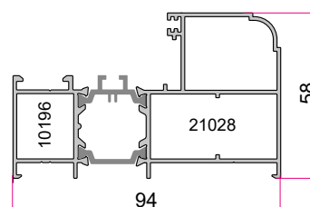
فریم کتیبه 94 Engraving Profiles 1.600 kg/m
