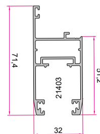
لنگه زهوار خور Sash 0.885 (kg/m)
