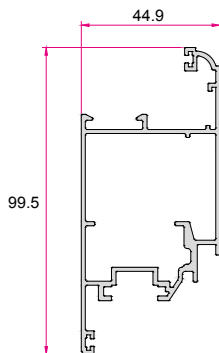
لنگه درب یراق پی وی سی خور Door Sash with PVC Fitting 1.330 (kg/m)
