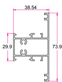
وادار وسط Heavy Duty Tripetalous 0.910 (kg/m)
