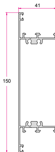
وادر وسط ۱۵ سانتی Tripetalous 1.765 (kg/m)
