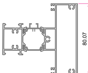
وادر کتیبه 94 Tripetalus 94 kg/m 2.320
