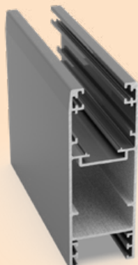
چهارچوب کشویی پهن یک طرف قوس Wide Sliding Frame 1.460 (kg/m)
