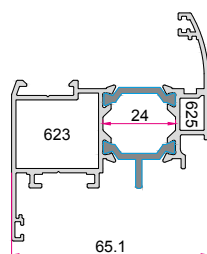
لنگه پنجره سری B Series "B" Window Sash 1.450 (kg/m)
