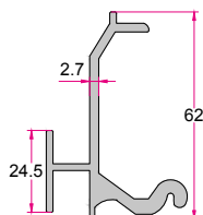
ریل سکوریت Security Glass's Rail 1.200 (kg/m)
