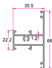
وادار مونوریل Tripetalous 0.650 (kg/m)
