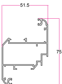
لنگه لولایی پنجره Window Sash 0.980 (kg/m)
