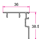
نبشی یک لبه Cap 0.320 (kg/m)
