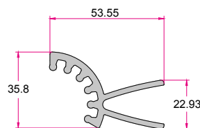
پروفیل چرخشی لوور مخصوص ۱۲۰۱ Louvre Adjustable Profile 1.050 (kg/m)
