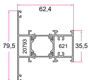
وادرلیفت اند اسلاید Tripetalous Profiles 1.550 kg/m
