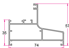
چهارچوب کتیبه ۷۴ Big Frame 0.930 (kg/m)
