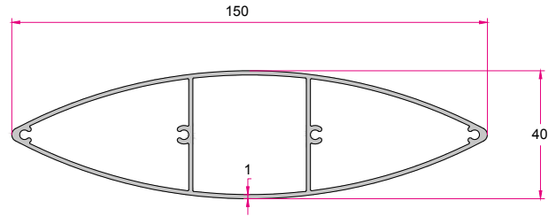
لوور ۱۵ 15cm Oval Louvre 1.690 (kg/m)
