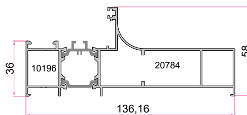
کتیبه لیفت اند اسلاید مونوریل سری ۱۳۶ و ۱۴۰ Engraring Profiles 1.750 kg/m
