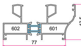
چهارچوب کشویی با ریل توری Sliding Frame with Fly Screen Rail 1.350 (kg/m)
