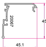
درپوش Cap 0.417 (kg/m)
