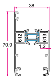
لنگه کشویی زهوارخور Sliding Sash 1.070 (kg/m)
