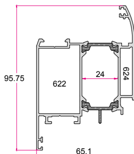
لنگه درب سری B Series "B" Door Sash 1.750 (kg/m)
