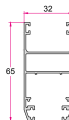
لنگه کشویی ساده سبک Light Simple Sliding Sash 0.800 (kg/m)
