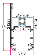
لنگه کشویی زهوارخور Sliding Sash 1.380 (kg/m)
