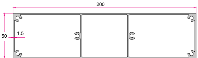
لوور ۲۰ 20cm Rectavngle Louvre 2.920 (kg/m)
