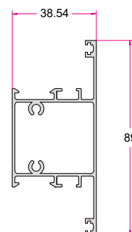
وادار وسط بزرگ Big Middle Tripetalous 0.985 (kg/m)
