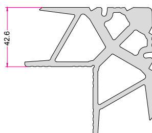
فیکس پانچی ۴۲ سنگین Corner Joint 5.440 (kg/m)
