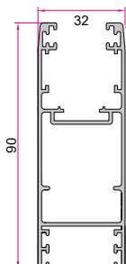
لنگه کشویی ساده کیپر دار ۹۰ 90mm Simple Sliding Sash 1.358 (kg/m)
