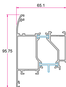
لنگه درب بیرون بازشو Outside Opening Door Sash 1.750 (kg/m)
