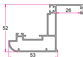
فریم‌لس دوجداره بازشو Double Glazed Opening Profile 1.050 (kg/m)
