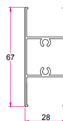
وادار وسط کشویی سری ۵۵ Series 55 Sliding Mullion 0.680 (kg/m)
