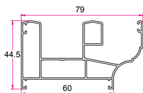
چهارچوب کشویی طرح‌دار Sliding Frame 1.060 (kg/m)
