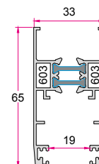
لنگه کشویی Sliding Sash 1.050 (kg/m)
