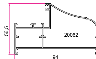
کتیبه نرمال ۹۴ Door Frame 1.280 (kg/m)
