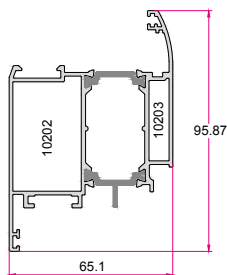
لنگه درب TH60 Big Door Sash 1.800 (kg/m)
