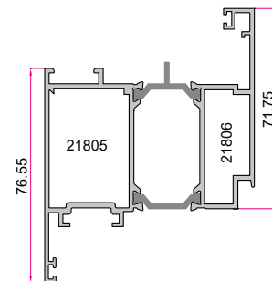
لنگه درب داخل بازشو Inside Opening Door Sash 2.330 (kg/m)
