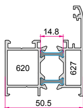
فریم کوچک سری A Series "A" Small Frame 1.300 (kg/m)
