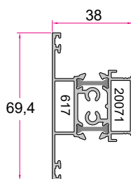
سپری برای لنگه کشویی T profile 1.050 kg/m
