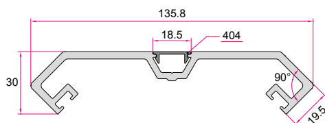
کنج بیرونی 90° Outer Corner Profiles 90° 2.252 (kg/m)
