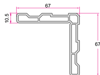
گونای ۱۰ سبک Corner Joint 1.520 (kg/m)
