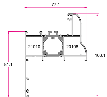
TH60 چهارچوب درب روکوب دار Door Frame 1.730 (kg/m)
