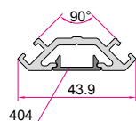
زهوار کنج داخلی Inner Corner Rickety 0.475 (kg/m)
