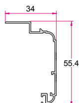
روکوب اختصاصی ۵ سانتیمتری casing 0.360 (kg/m)
