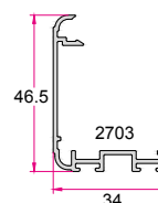
درپوش لنگه Cap 0.390 (kg/m)
