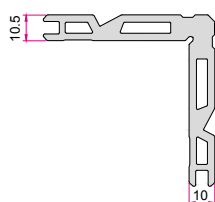
فیکس پانچی ۱۰ Corner Joint 2.450 (kg/m)
