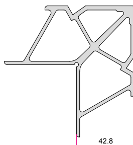
فیکس پانچی ۴۲ سبک Corner Joint 3.479 (kg/m)
