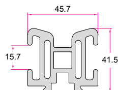
لقمه افقی Sliding Piece 2.340 (kg/m)
