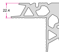
فیکس پانچی ۲۲ Corner Joint 3.700 (kg/m)
