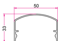
درپوش کرو عمودی ۳۳ Mullion Curved Cap 0.427 (kg/m)
