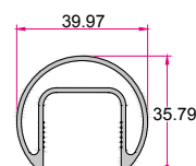
شیشه گیر بالا Handrail 0.840 (kg/m)
