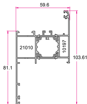
TH60 چهارچوب پنجره روکوب دار Window Frame 1.450 (kg/m)
