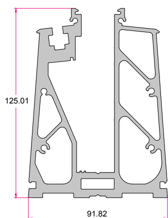
شیشه گیر پایین Mounting Bracket 7.830 (kg/m)
