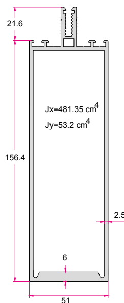
پروفیل شیشه خور ۲۱/۶ یو-چنل U-Channel Profile 3.780 (kg/m)
