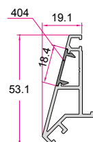
آداپتور کنج داخلی 90° Inner Corner Adaptor 90° 0.535 (kg/m)
