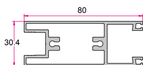
عرض بالا و پایین Top and Bottom Profile 1.440 (kg/m)
