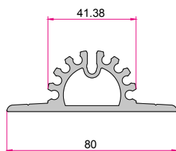
پایه لوور Louvre Base Profile 1.458 (kg/m)
