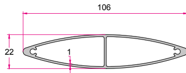
لوور ۱۰ 10cm Oval Louvre 0.930 (kg/m)
