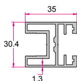
عمودی ۳ سانتی Side Rail 0.775 (kg/m)
