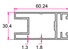
عمودی ۶ سانتی Side Rail 1.040 (kg/m)
