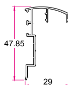
نبشی یک لبه ساده سری ۵۵ برای قالب‌های ۱۲۲ و ۱۲۸ Cap 0.360 (kg/m)
