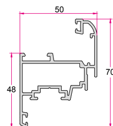
لنگه پنجره Window Sash 1.160 (kg/m)
