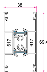
وادر بدون زهوار Tripetalous 1.278 (kg/m)
