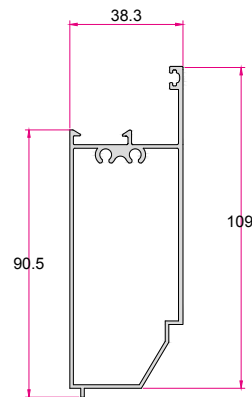
پروفیل پاخور درب Bottom Door Sash 1.100 (kg/m)
