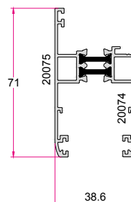
لنگه زهوار خور Sliding Sash 1.060 (kg/m)
