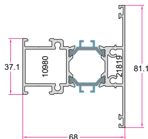
وادر Door Sash 1.800 (kg/m)
