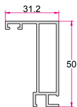
فریم بازشو Opening Frame 0.665 (kg/m)
