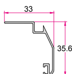
روکوب اختصاصی ۳ سانتیمتری casing 0.220 (kg/m)
