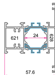
سپری سری B Series "B" Tripetalous 1.500 (kg/m)
