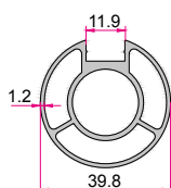
لوله ۴۰ Pipe 40 0.900 (kg/m)
