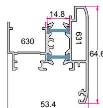
وسط دولنگه سری A Series "A" Middle Sash 1.200 (kg/m)
