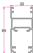
لنگه کشویی طرح دار کیپر خور Sliding Sash 0.870 (kg/m)
