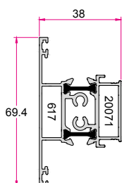
وادر زهوار خور Tripetalus 1.102 (kg/m)
