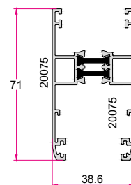
لنگه بدون زهوار Sliding Sash 1.180 (kg/m)
