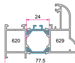
فریم بزرگ سری B Series "B" Big Frame 1.600 (kg/m)
