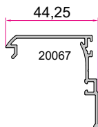
اینترلاک Inter Lock For Sliding Vent 0.436 kg/m
