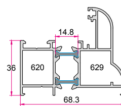
فریم بزرگ سری A Series "A" Big Frame 1.500 (kg/m)
