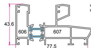
چهارچوب کشویی سنگین Heavy Duty Sliding Frame 1.650 (kg/m)
