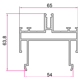
پروفیل افقی Transom 1.590 (kg/m)
