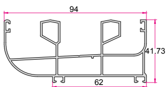
چهارچوب کشویی پهن یک طرف قوس لاستیک خور Wide Sliding Frame with Rubber Place 1.460 (kg/m)
