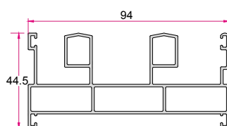
چهارچوب کشویی پهن Wide Sliding Frame 1.600 (kg/m)
