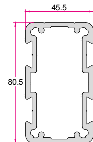
پروفیل اتصال ۱۱۰۲ Connector 2.573 (kg/m)
